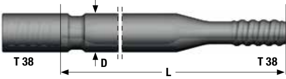
Female end OD 56 mm
